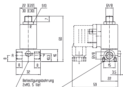
Ausführung mit Gewindeanschluss G 1/8
